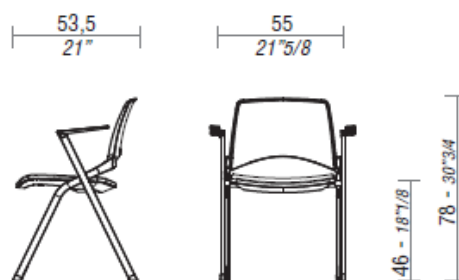
KENDO, sedia con braccioli.
