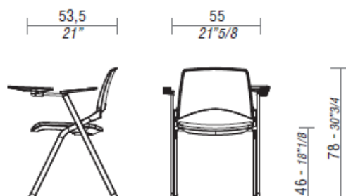
KENDO, sedia con tavoletta.
